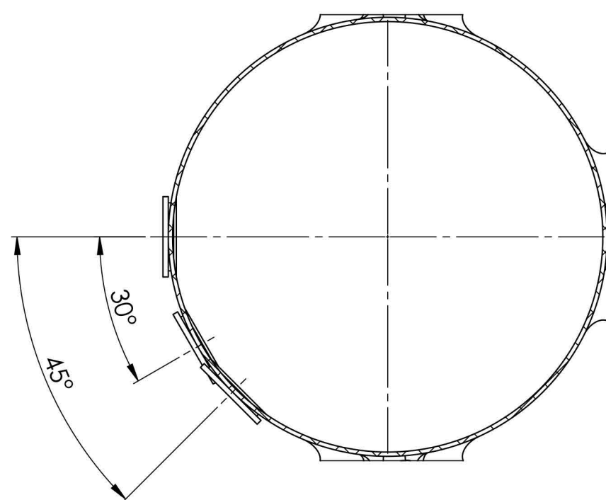
A-A (1 : 10)
