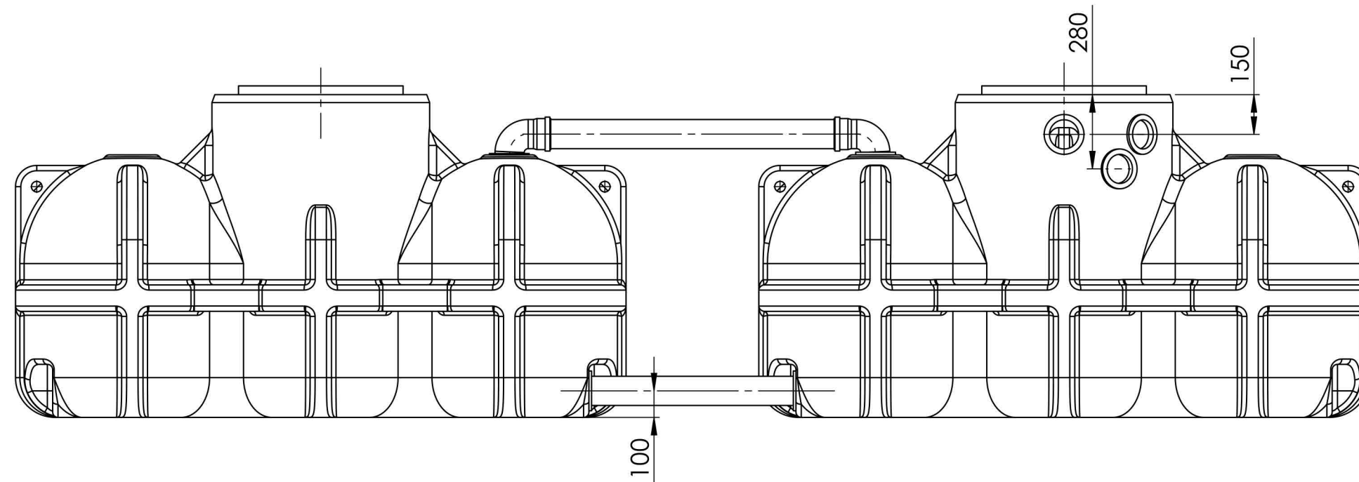
A-A (1 : 10)
